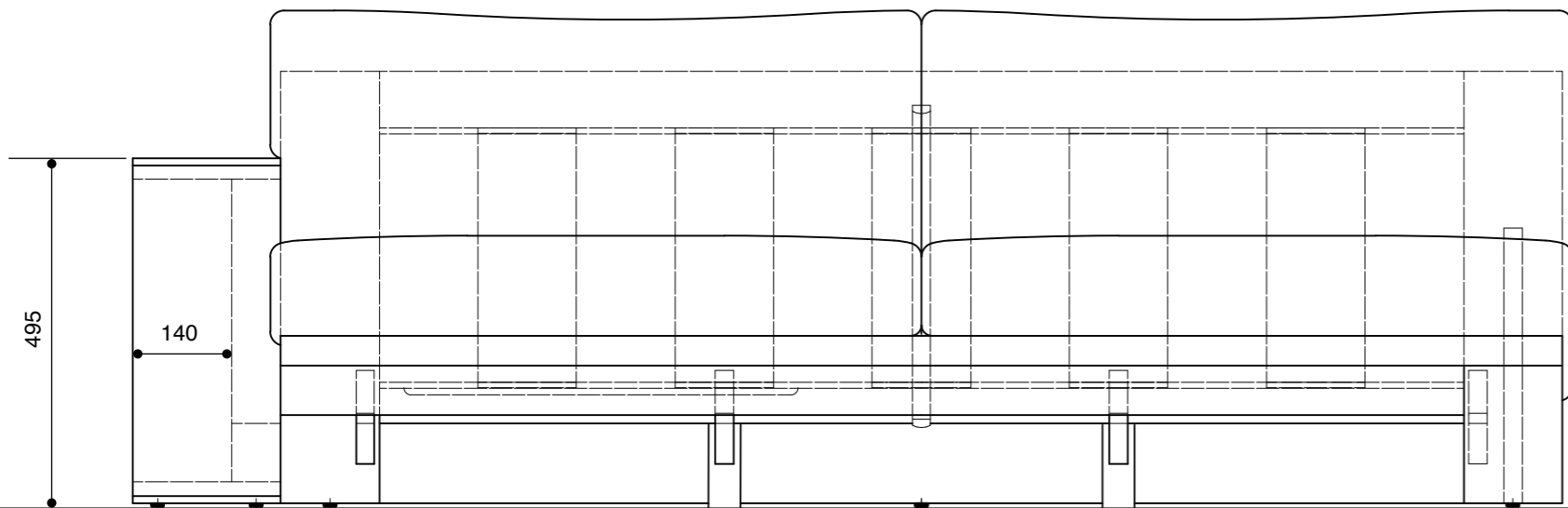
【正面】
