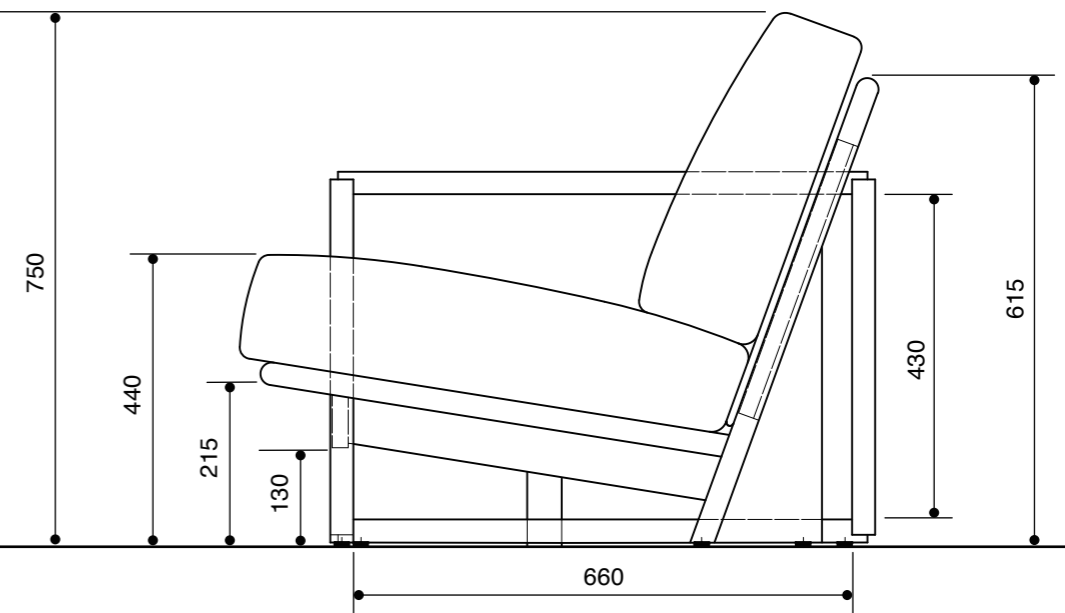
【側面】
