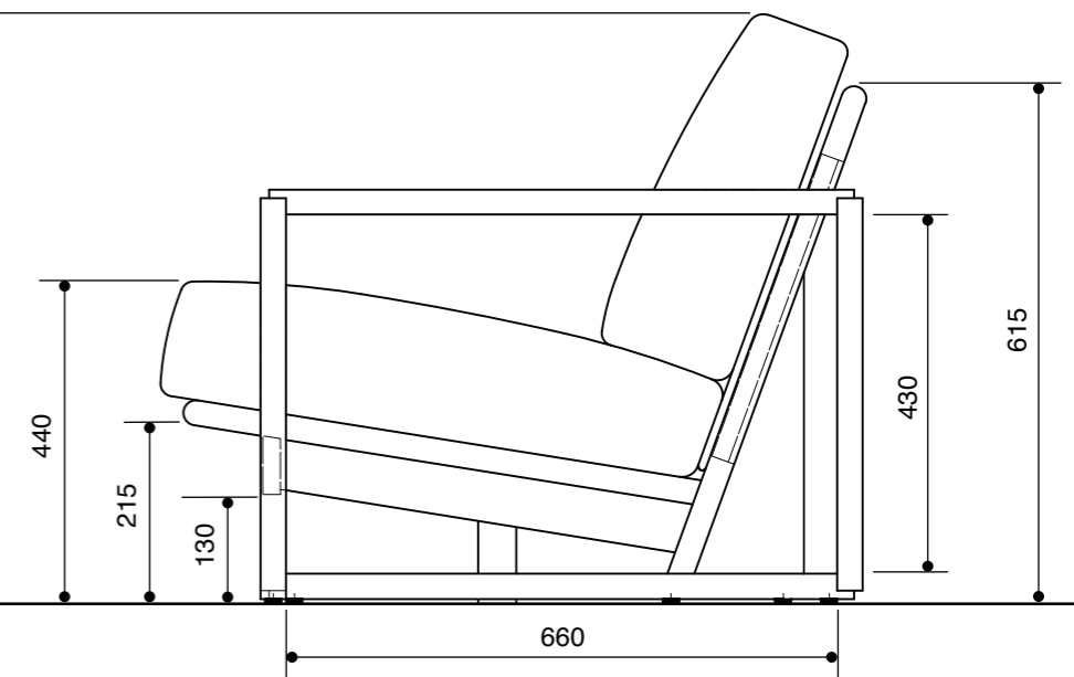
【側面】
