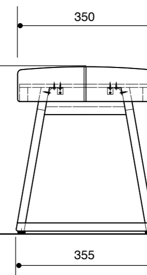
【側面】
