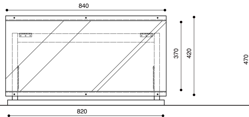
【正面】
