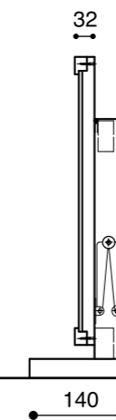
【側面】
