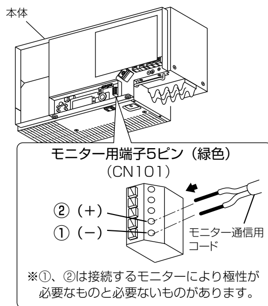
モニター通信用コードの接続箇所
