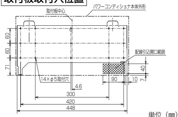
取付板取付穴位置
