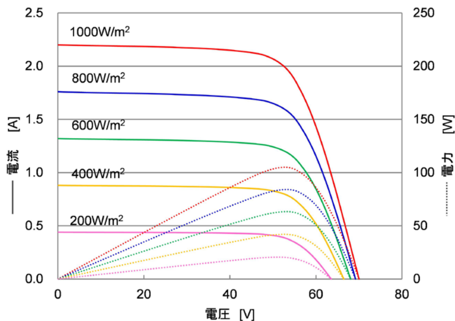
放射照度別 I-V P-V 代表特性 型式:SFR105-A 測定条件:AM1.5 25°C
