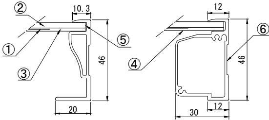
SECTION A-A(A-A 断面)
