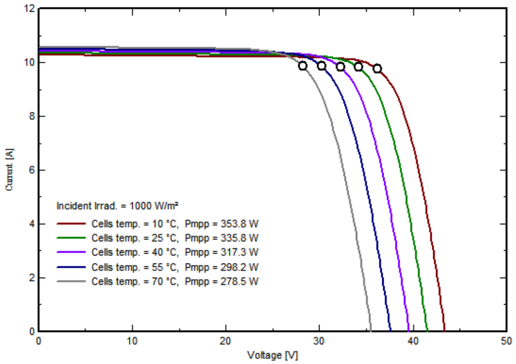
PV module: Jinkosolar, JKM 335M-60H
