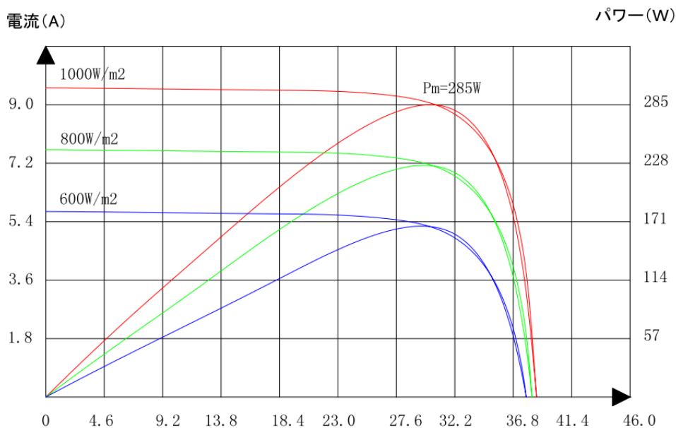
電流・電圧とパワー・電圧カーブ(285W)
