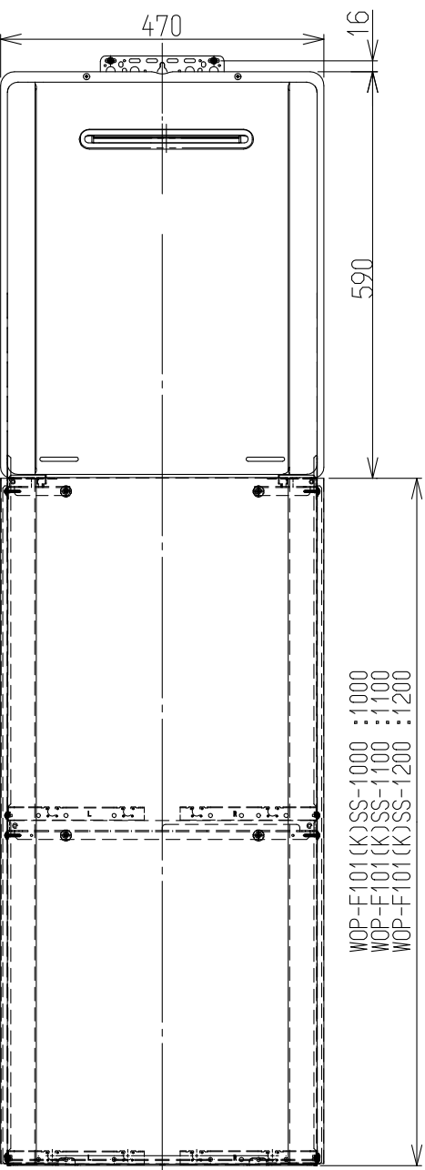
配管カバー取付図(1:10)
