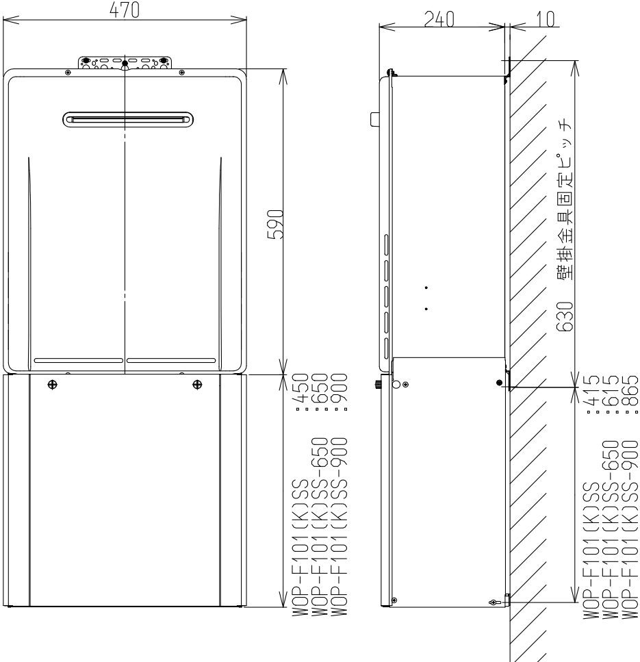
配管カバー取付図(1:10)
