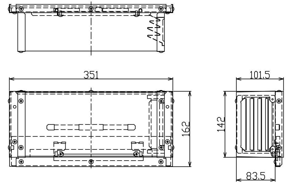
側方排気アダプタ寸法図
