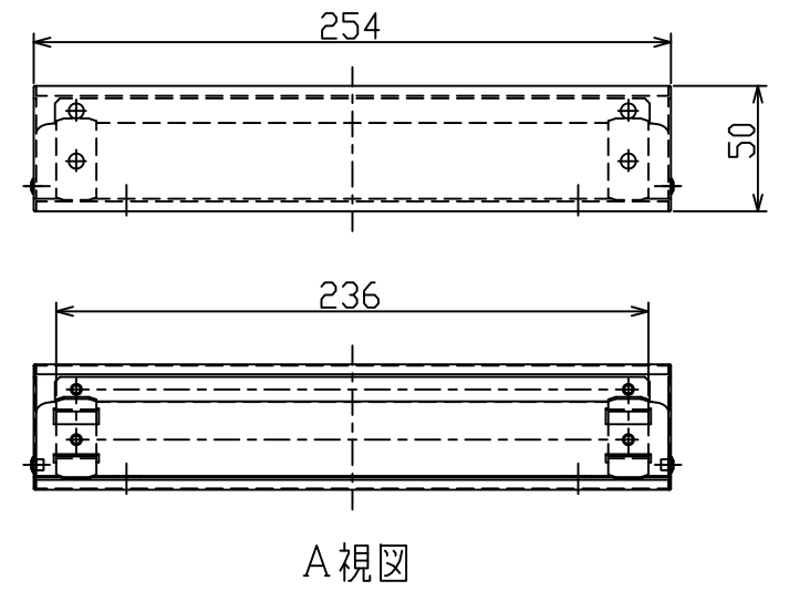
排気カバー寸法図
