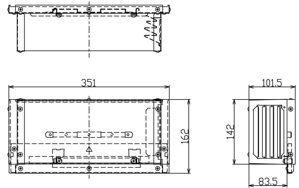
側方排気アダプタ寸法図
