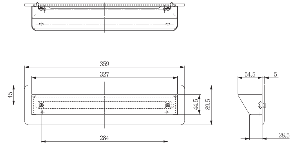
排気カバー寸法図
