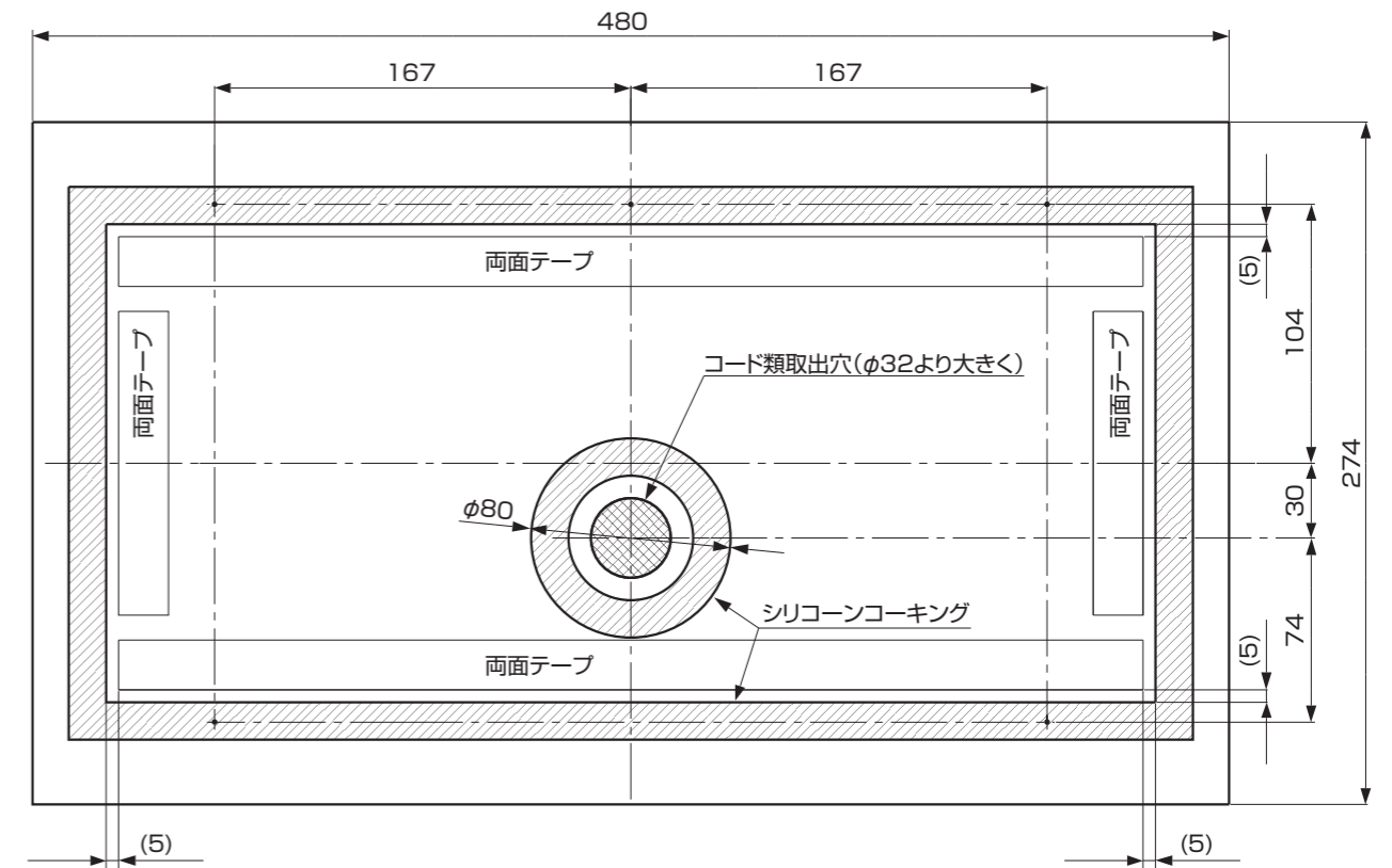
DSP-1600 化粧プレート裏面図 (単位:mm)
