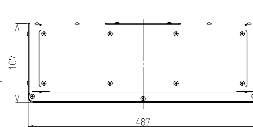
側方排気アダプタ寸法図
