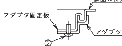
B部取付模式図(上から見た図) 機器の排気口
