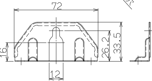
●取付金具下詳細図 (S=1:2) 左右共通
