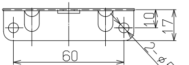
●取付金具上詳細図 (S=1:2)
