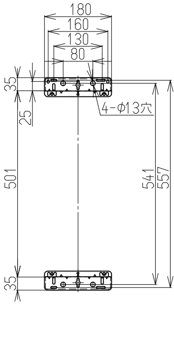
●取付金具下詳細図 (S=1:2) 左右共通
