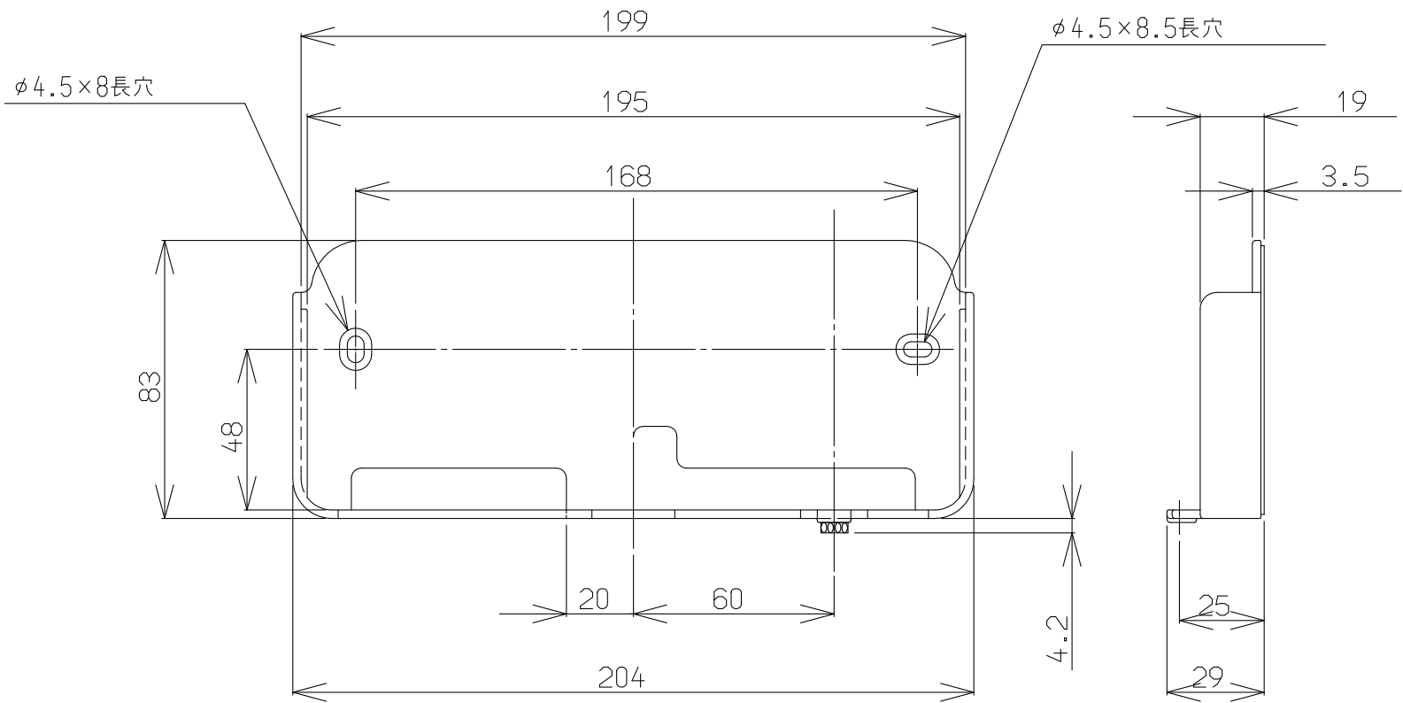
浴室リモコン取付板
