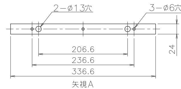
■配管カバー下後板 壁面取付ピッチ
