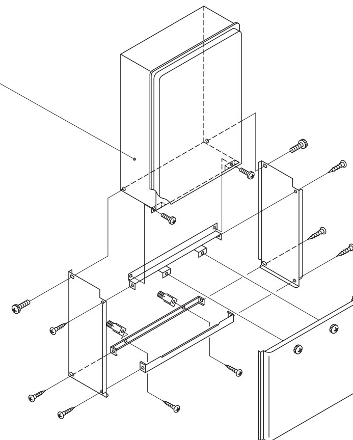
■組立図（概略）
