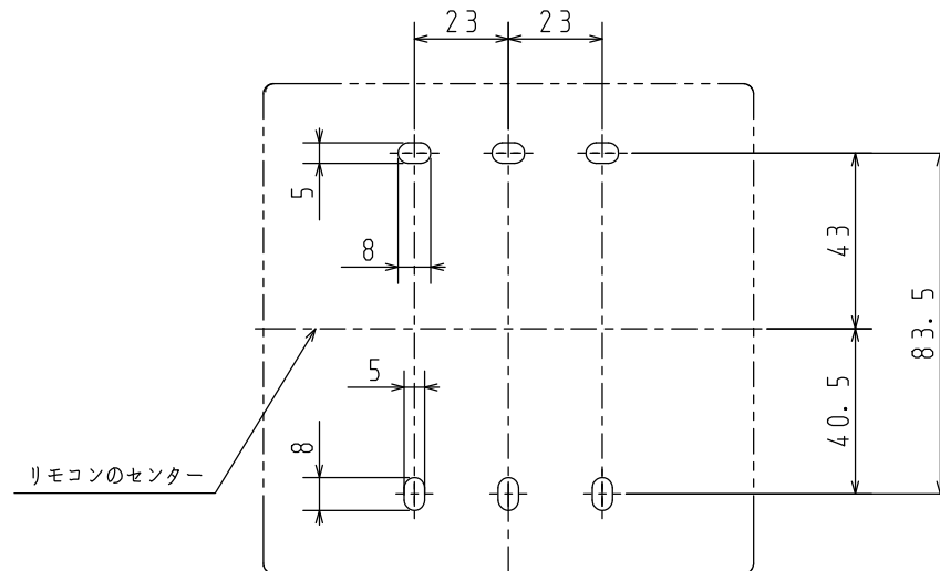
取付寸法
