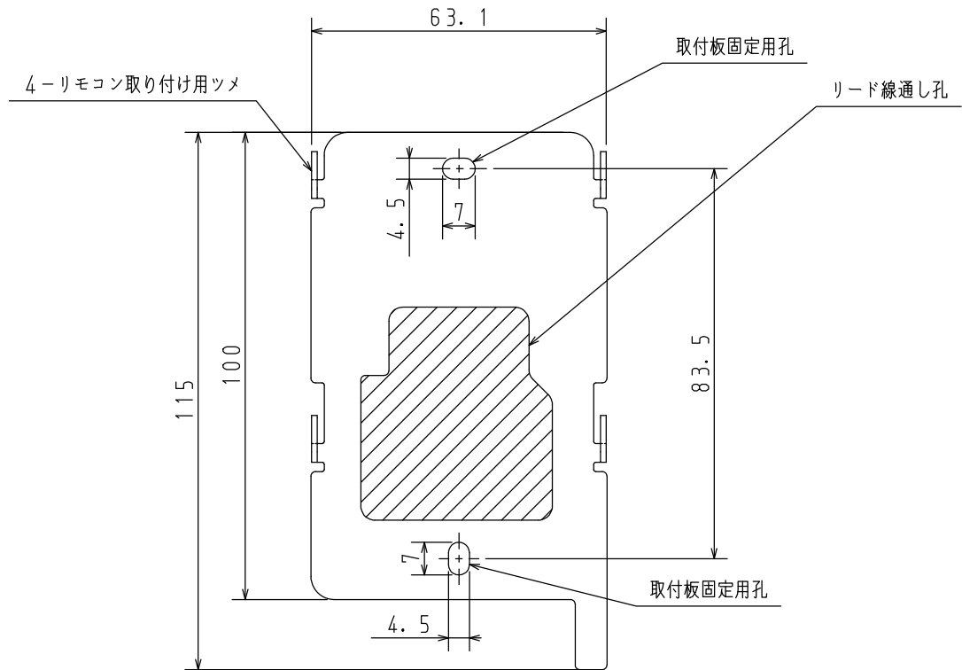
取付板図 t 1.2 正面から見た位置
