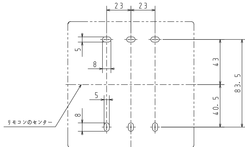
取付寸法
