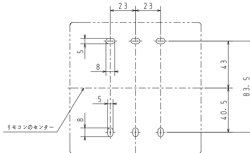
取付寸法
