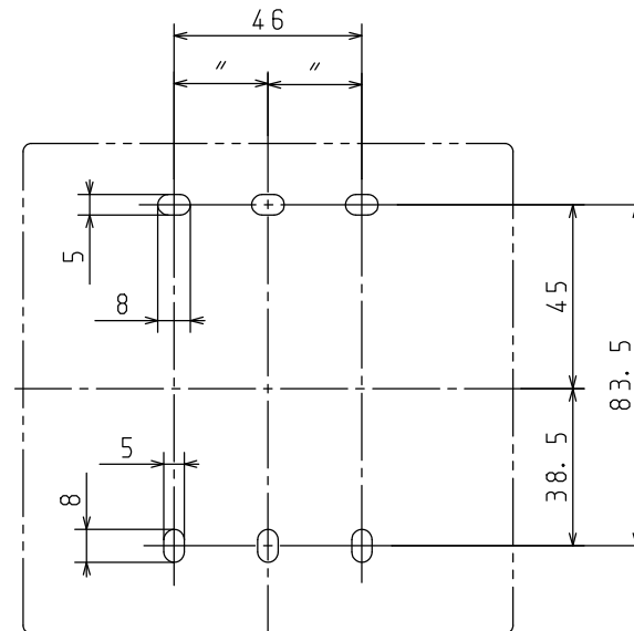
取付寸法 正面から見た位置
