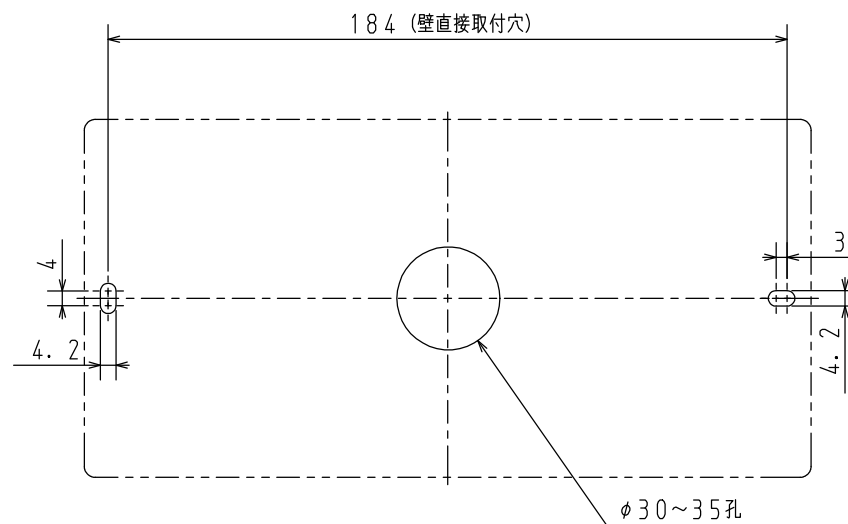
取付寸法 正面から見た位置
