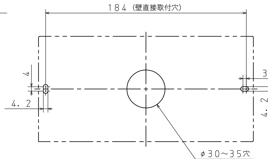
取付け寸法 正面から見た位置
