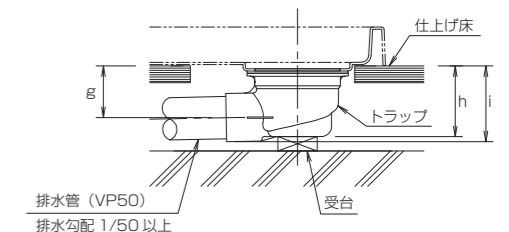
TP-52、TP-54 の場合
