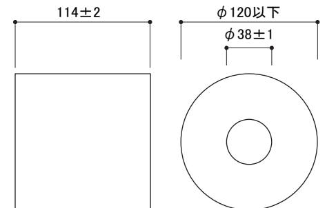
推奨するトイレットペーパーの寸法(JIS規格)
