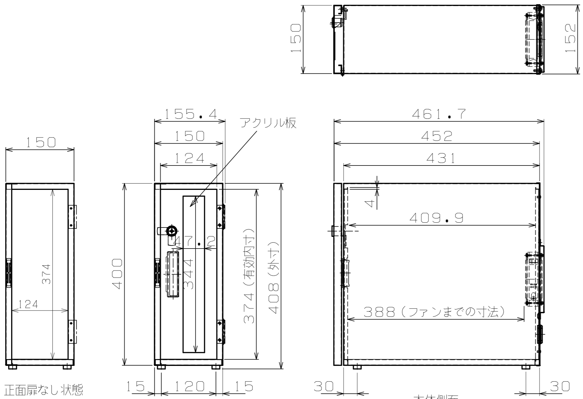
本体正面
