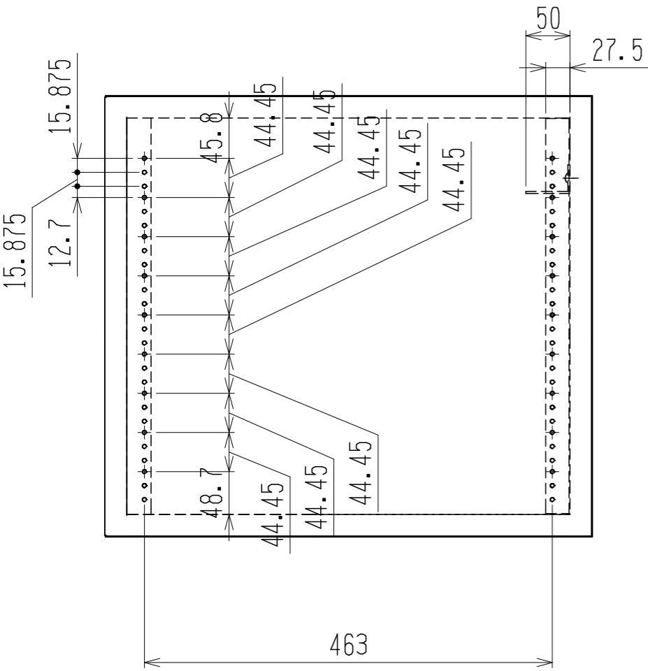
オプション・19インチ用穴寸法
