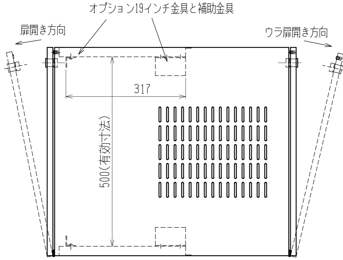
固定ベルト 取り付け位置 (上から見た図)
