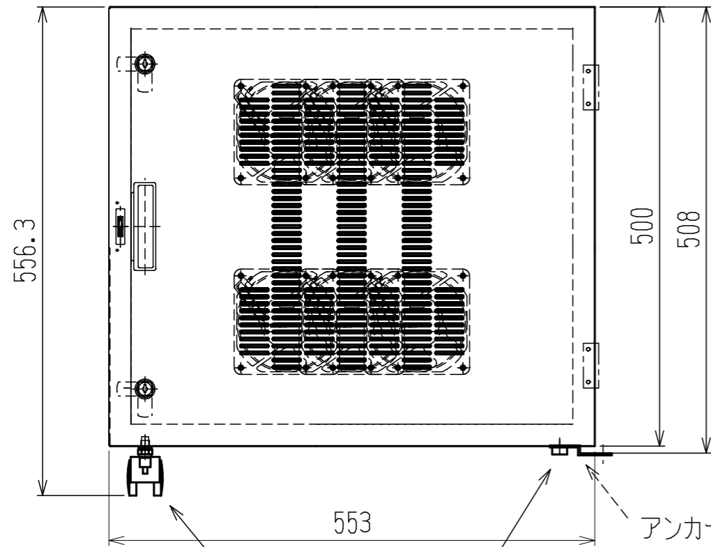
キャスターを組み付けた場合
