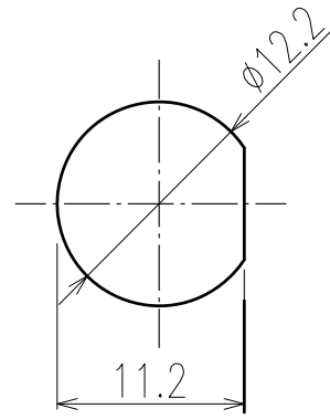
取付穴参考寸法図
