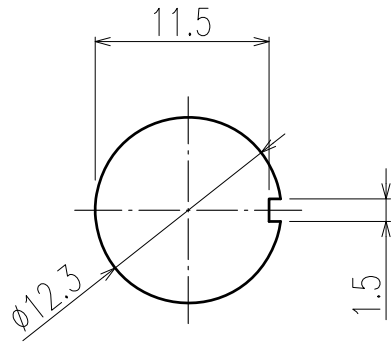
取付穴参考寸法図
