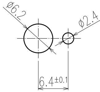
取付穴参考寸法図
