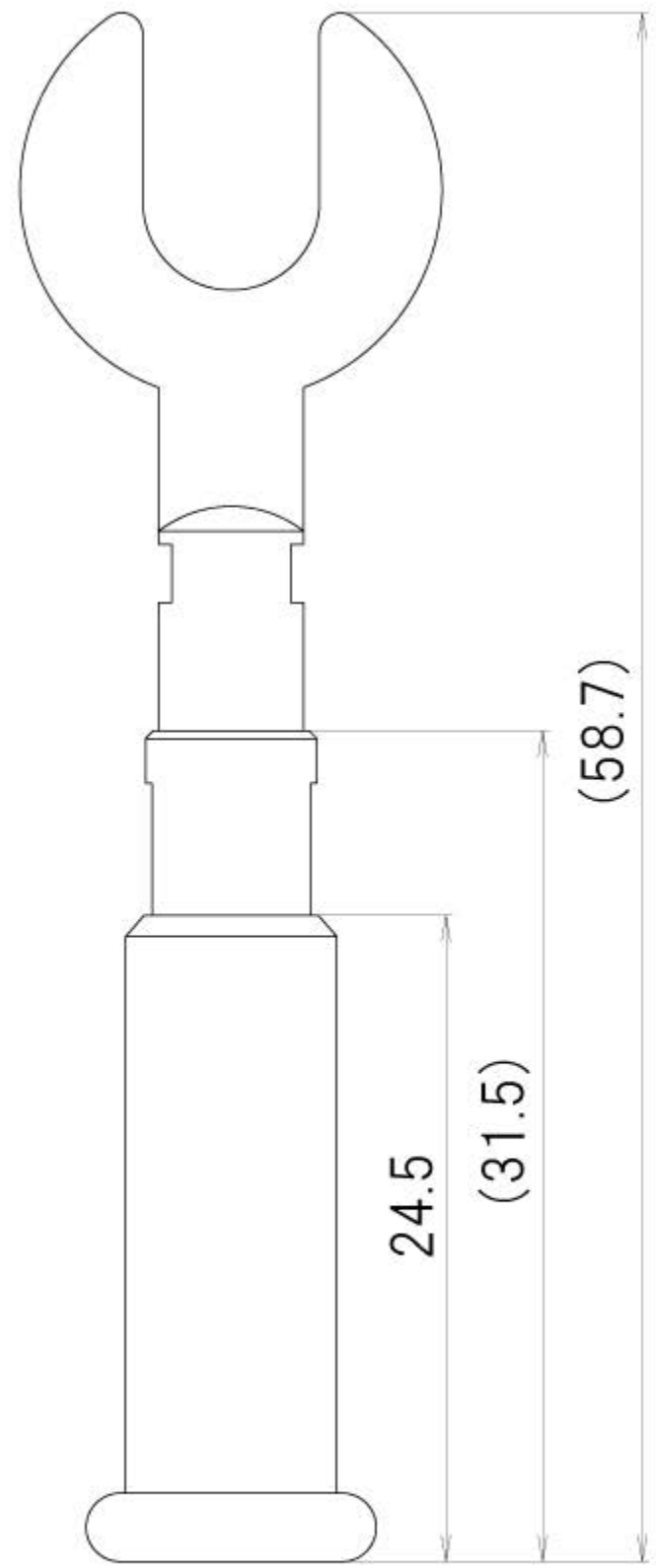
TJ-100+TJ-100-KA 組み合わせ状態
