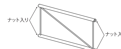
⑥背補強×1
