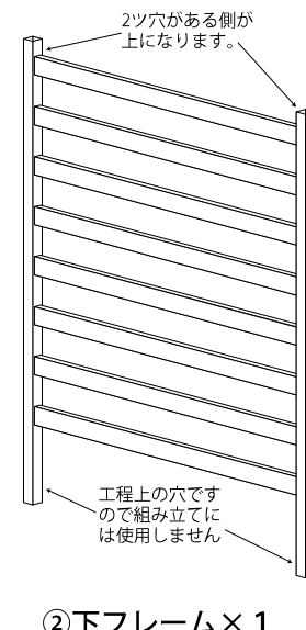
②下フレーム×1
