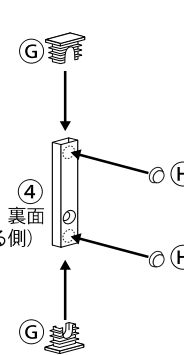
※2セット組み立てます。
