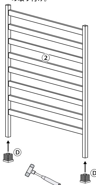
※2セット組み立てます。
