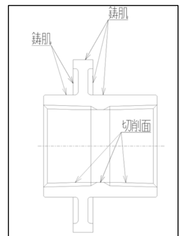
外観図示
