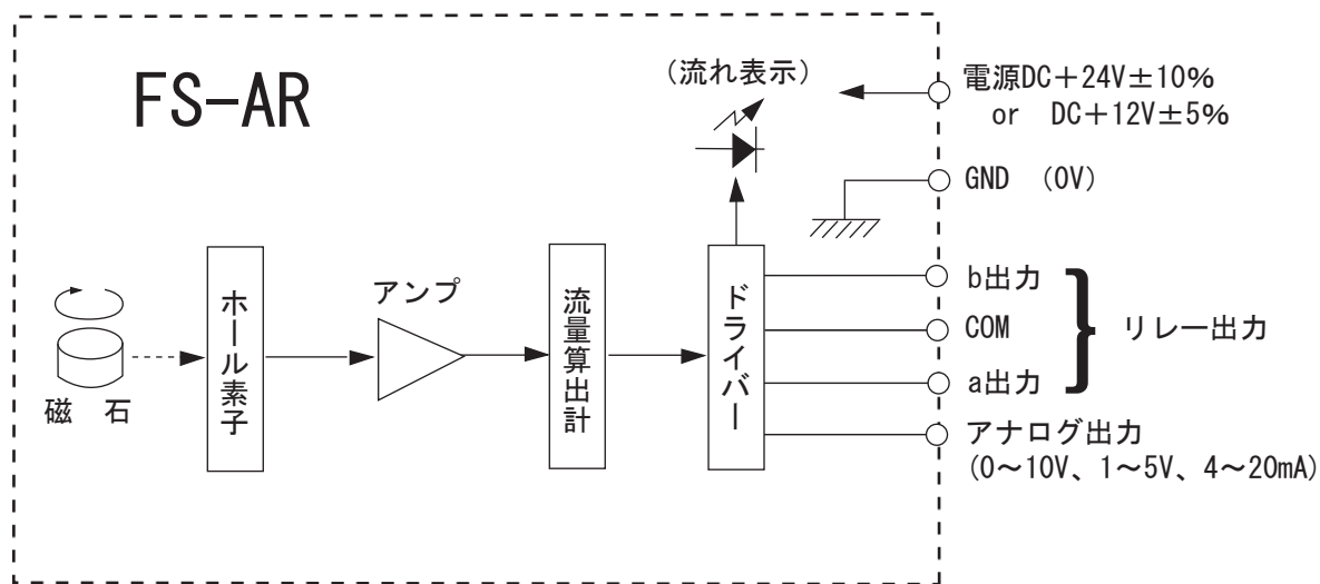
FS-ARブロック図
