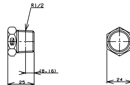
TITLE 六角プラグ(テーパ-ねじ) MODEL R-8-1/2
