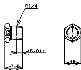
TITLE 六角プラグ(テーパ-ねじ) MODEL R-8-1/4
