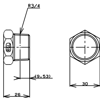
TITLE 六角プラグ(テーパ-ねじ) MODEL R-8-3/4
