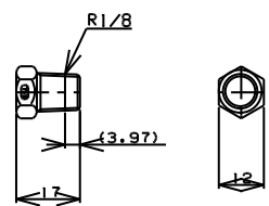
TITLE 六角プラグ(テーパ-ねじ) MODEL R-8-1/8
