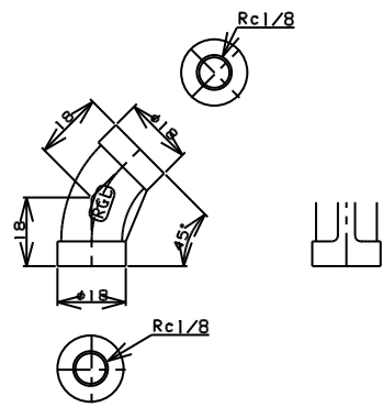
TITLE 45° エルボ MODEL R-5-1/8
