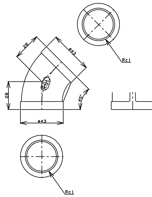
TITLE 45° エルボ MODEL R-5-1
