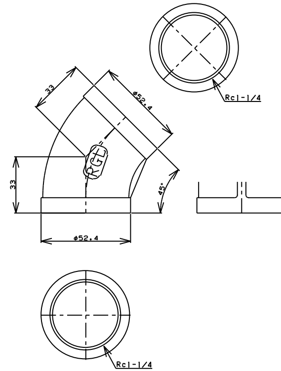
TITLE 45° エルボ MODEL R-5-1-1/4
