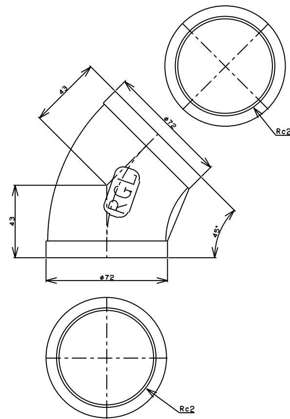
TITLE 45° エルボ MODEL R-5-3/4
