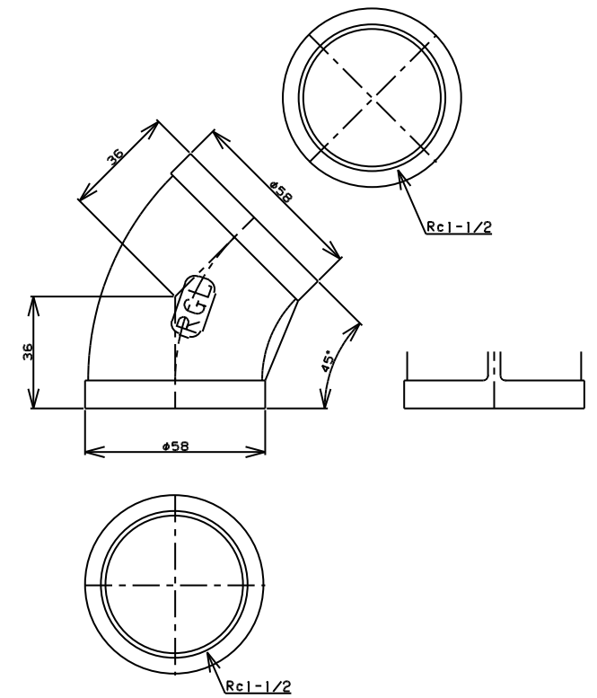
TITLE 45° エルボ MODEL R-5-1-1/2
