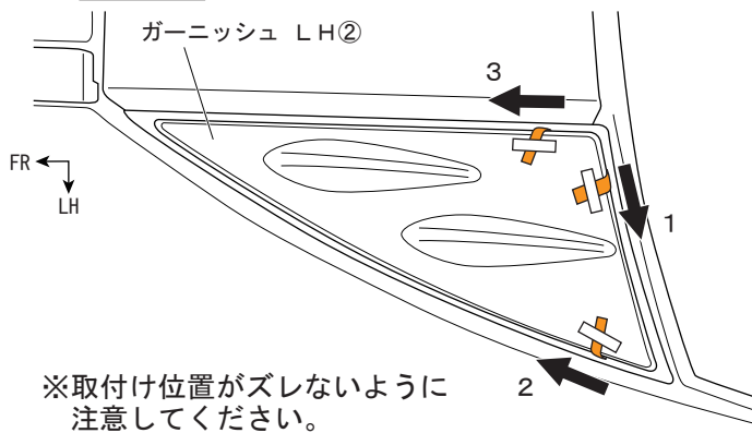
図7 上面視 ※LH図示 左右共通作業
