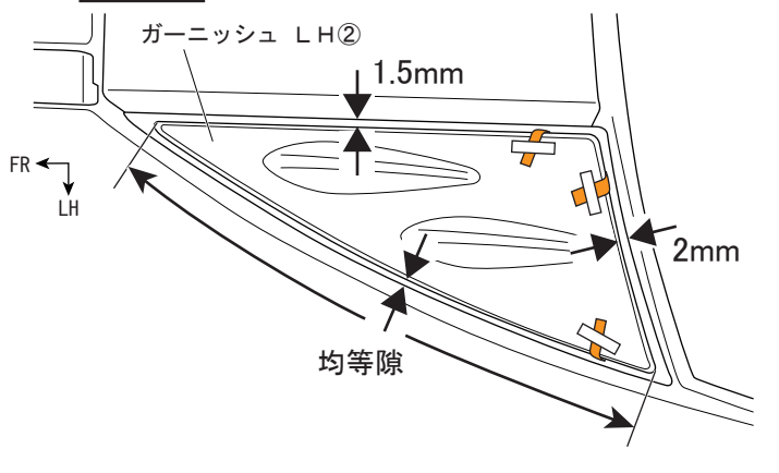
図6 上面視 ※LH図示 左右共通作業
