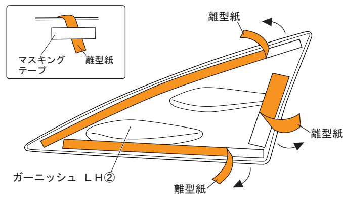
図5 裏面視 ※LH図示 左右共通作業
