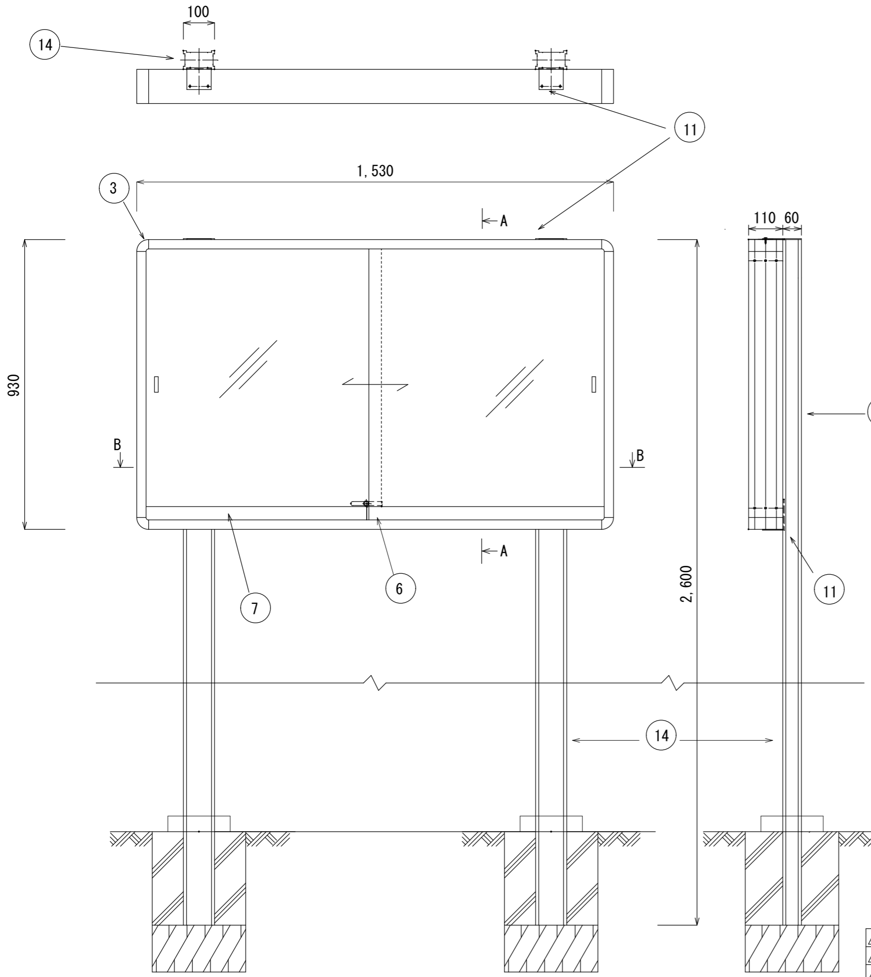
D-110 1530×930自立 シリンダー錠
