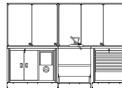
Banco per lavoro su sospensioni e motori con vasca e piano INOX dotato di griglie INOX sulla vasca e sul piano di lavoro con arrotolatore aria compressa vasca estraibile raccogli olio sotto la morsa
