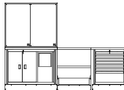
Banco per lavoro su sospensioni e motori con vasca e piano INOX dotato di griglia INOX sulla vasca e vaschetta estraibile raccogli olio sotto la morsa
