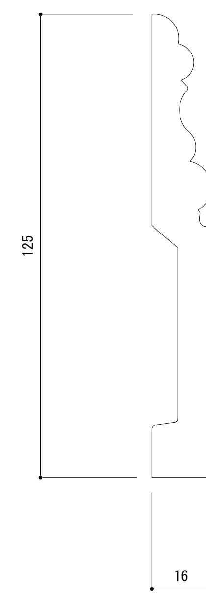
NMG098 125×16 ※ ポリウレタン製の為、若干の寸法誤差がある場合があります。
