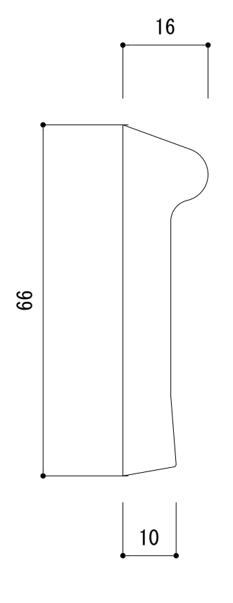
NMG067 66×16 ※ ポリウレタン製のため、若干の寸法誤差がある場合があります。
