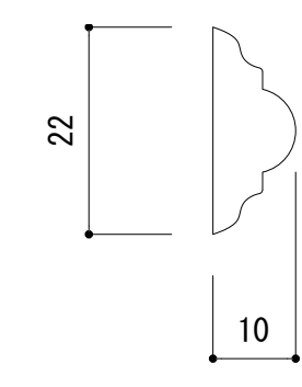
NMG102 22×10 ※ ポリウレタン製の為、若干の寸法誤差がある場合があります。
