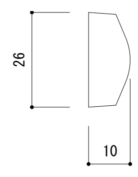
NMG092 26 × 10 ※ ポリウレタン製の為、若干の寸法誤差がある場合があります。
