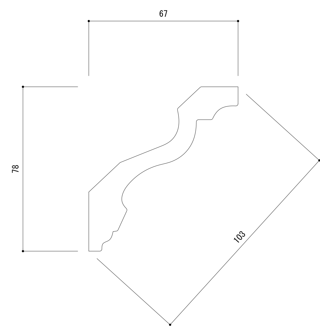
NMG010 78×67×100 ※ ポリウレタン製のため、若干の寸法誤差がある場合があります。
